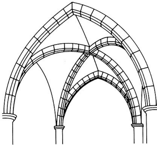
la voûte sur croisée d'ogives
